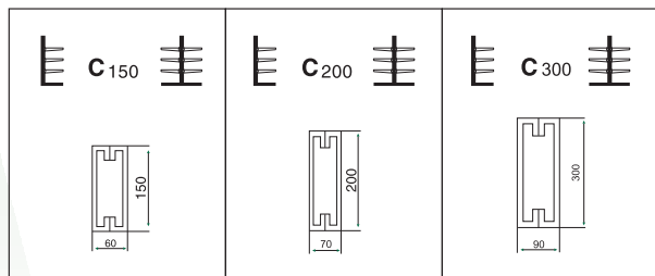
ВИДОВЕ КОЛОНИ POST SECTION SERIES
